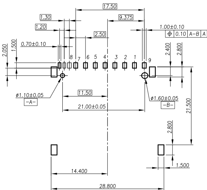
P.C.B Layout
