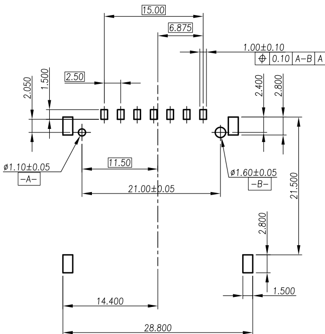
P.C.B Layout
